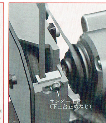
サンダー土台(下)
